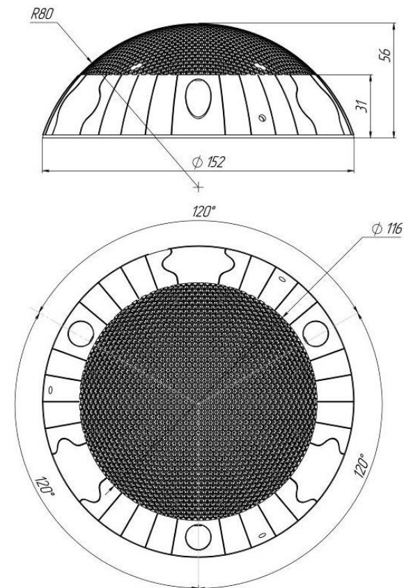
Рисунок 1 Светильник «Sveteco NEW 8»
