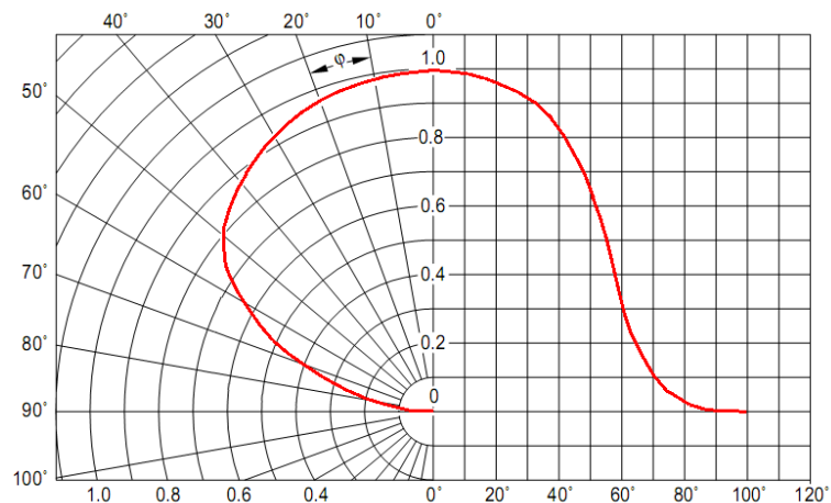
Рисунок 3 Тип КСС в исполнении «Д»
