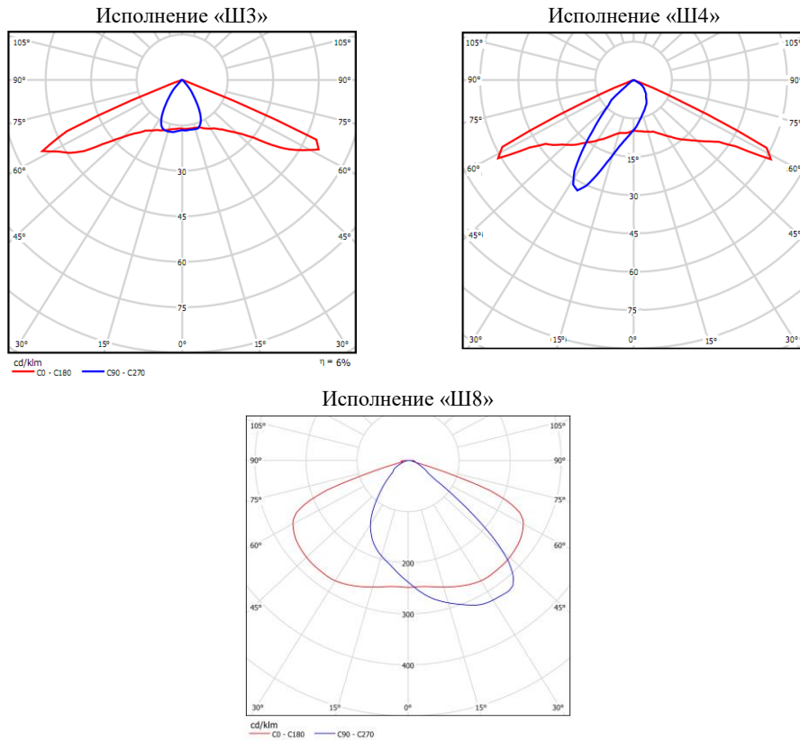
Рисунок 3 Типы КСС
