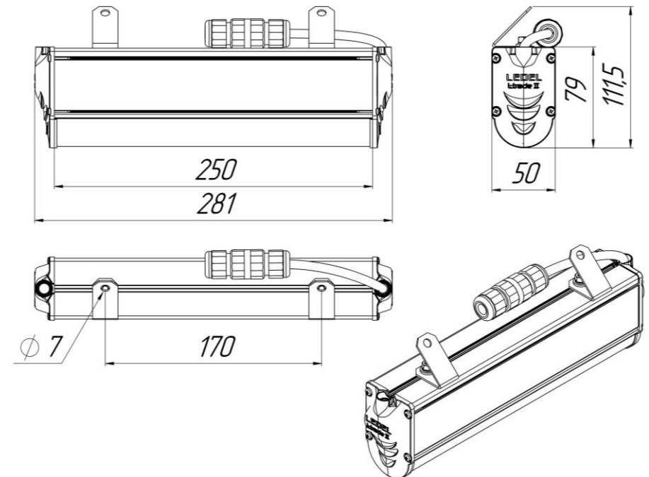
Рисунок 1 Светильник «L-trade II с фиксированным угловым креплением»
