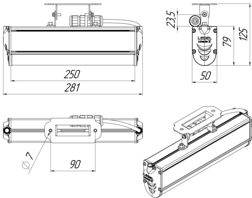
Рисунок 2 Светильник «L-trade II 12 с поворотным креплением»
