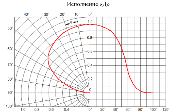
Рисунок 6 Тип КСС
