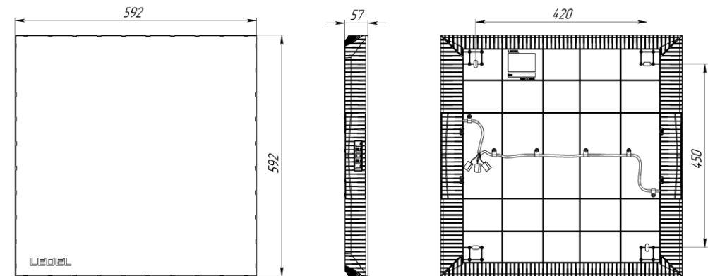
Рисунок 1 Светильник «L-office 55/Em»
